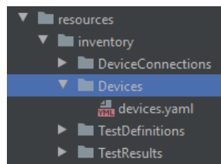
Abbildung 13: Position devices.yaml
