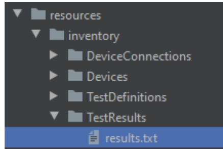
Abbildung 26: Position Testresultate
