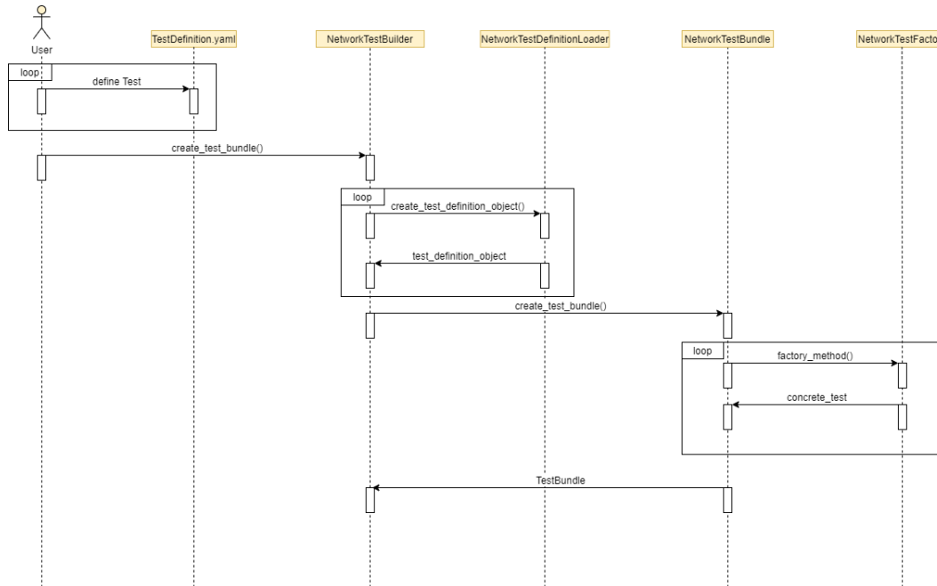
Abbildung 8: TestBundle Sequenzdiagramm
