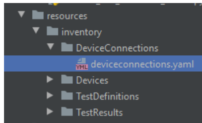
Abbildung 15: Position deviceconnections.yaml
